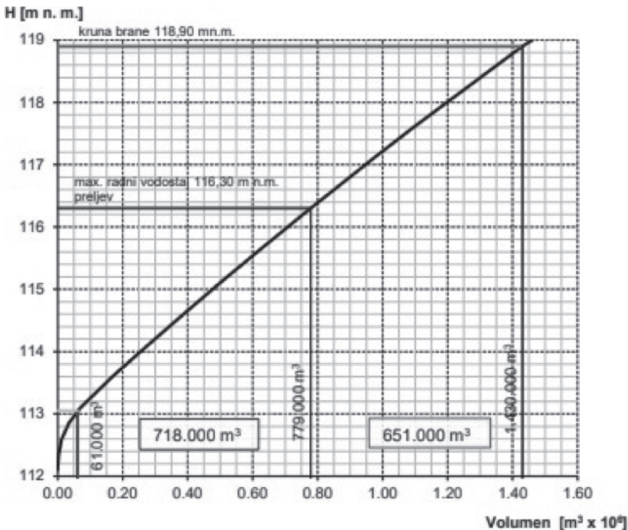
Slika 2. Krivulja volumena akumulacije
