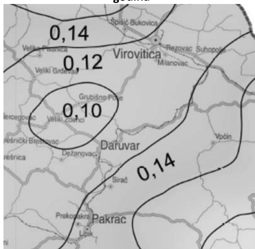
Slika 9. Vršna ubrzanja tla uzrokovana potresima za područje Općine Sirač, za povratni period 475 godina
