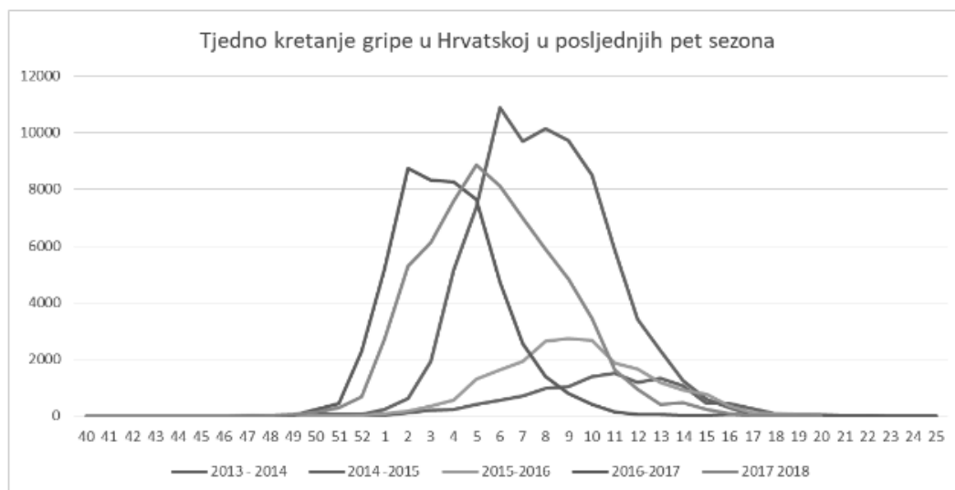
Grafikon 1. Tjedno kretanje gripe u RH u posljednjih pet sezona
