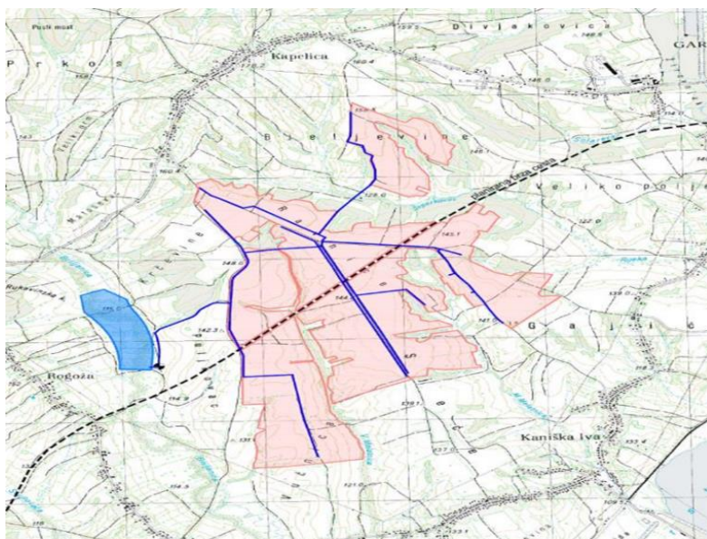
Slika 1. Situacija sustava navodnjavanja Kapelica - Kaniška Iva
