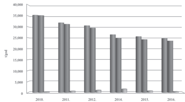
Graf 3. Ukupne količine otpada odložene na odlagališta u BBŽ u razdoblju od 2010. – 2016. godine
