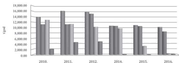
Graf 1. Ukupne količine prijavljenog proizvedenog neopasnog otpada na području županije u razdoblju od 2010. – 2016. godine
