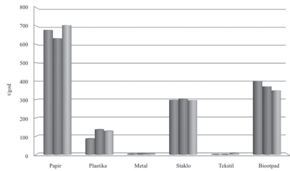
Graf 7. Količine odvojeno skupljenog otpada
