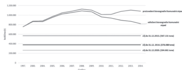
Slika 2. Proizvedeni i odloženi biorazgradivi komunalni otpad za razdoblje od 1997. do 2014. u odnosu na ciljane količine propisane Direktivom o odlaganju otpada
