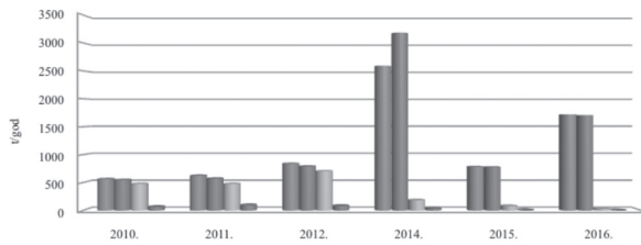
Graf 2. Ukupne količine prijavljenog proizvedenog opasnog otpada na području županije u razdoblju od 2010. – 2016. godine
