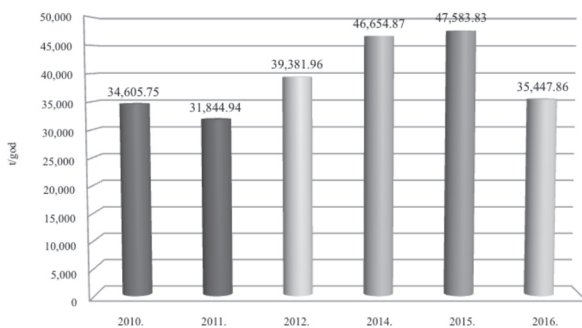
Graf 4. Ukupne količine otpada odložene u razdoblju od 2010. – 2016. godine po odlagalištu otpada
