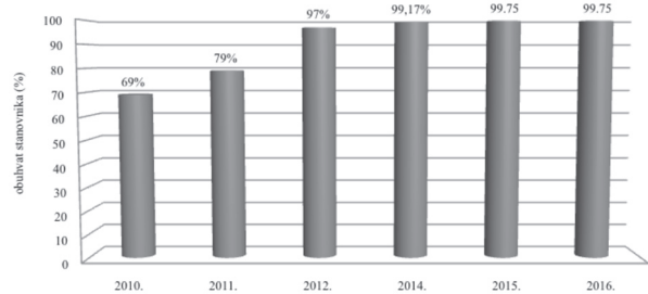
Graf 5. % stanovnika obuhvaćen organiziranim skupljanjem i odvozom komunalnog otpada u BBŽ
